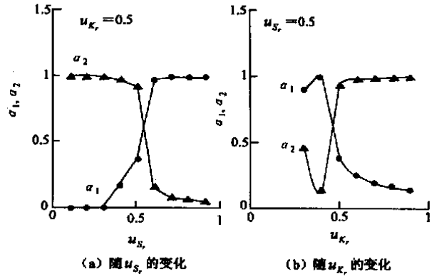
图1 敏感系数随 \mu_{S_r} 、 \mu_{K_r} 的变化
