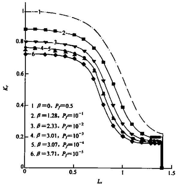
图 5 等可靠性指标线(R6 通用评定曲线)
