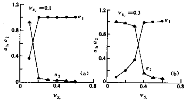
图2 敏感系数随 \nu_{S_r} 的变化
