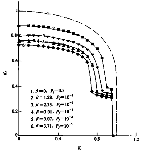
图 4 等可靠性指标线(PD6493 评定曲线)
